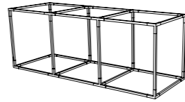
Y1-130 6500 x 2220 x 2400
